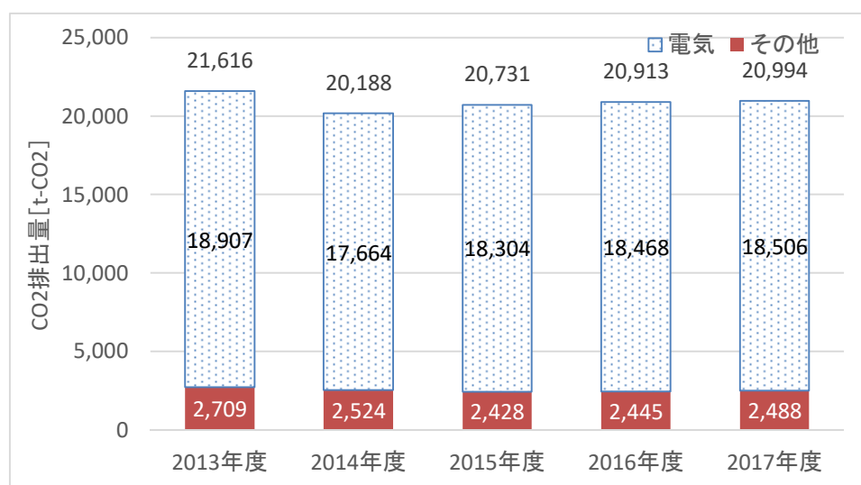
図 3-4 温室効果ガス排出量の推移（各施設 2013 年度の電気事業者基礎排出係数で算出）
