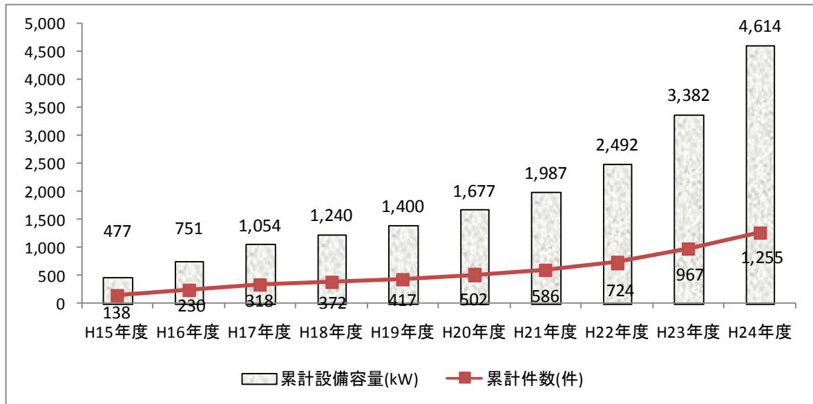
グラフ 6-5 太陽光発電システム設置件数の推移
