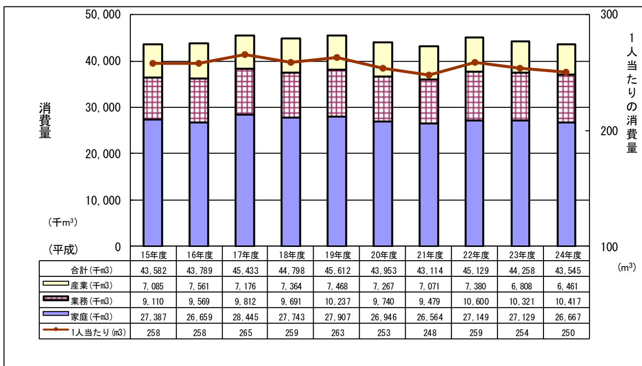
グラフ 6-7 用途別年間ガス消費量の推移
