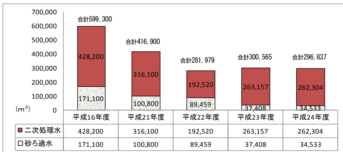
グラフ 6-3 七里ガ浜浄化センター処理水の再利用
