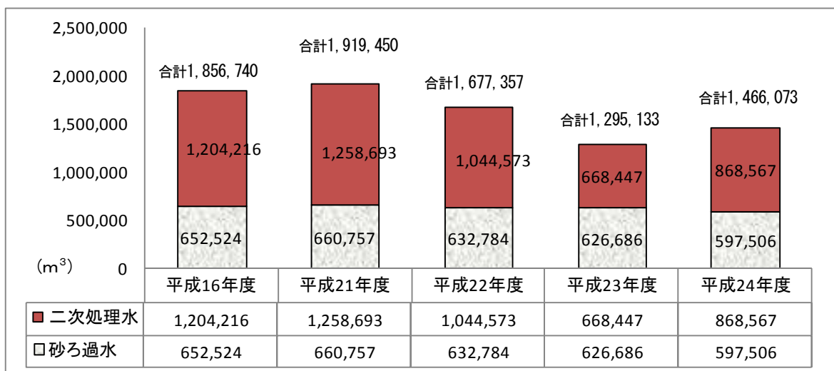
グラフ 6-4 山崎浄化センター処理水の再利用
