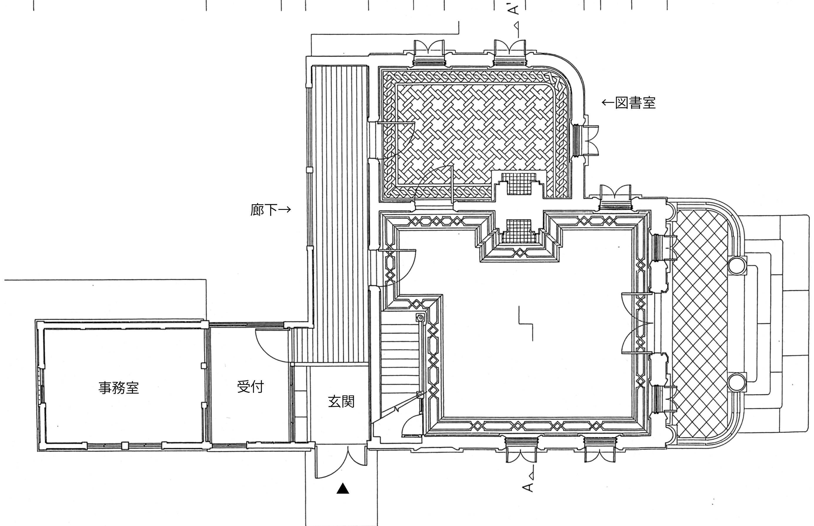
長谷子ども会館 1 階平面図 (文化財部分) (S=1/50(A3))
