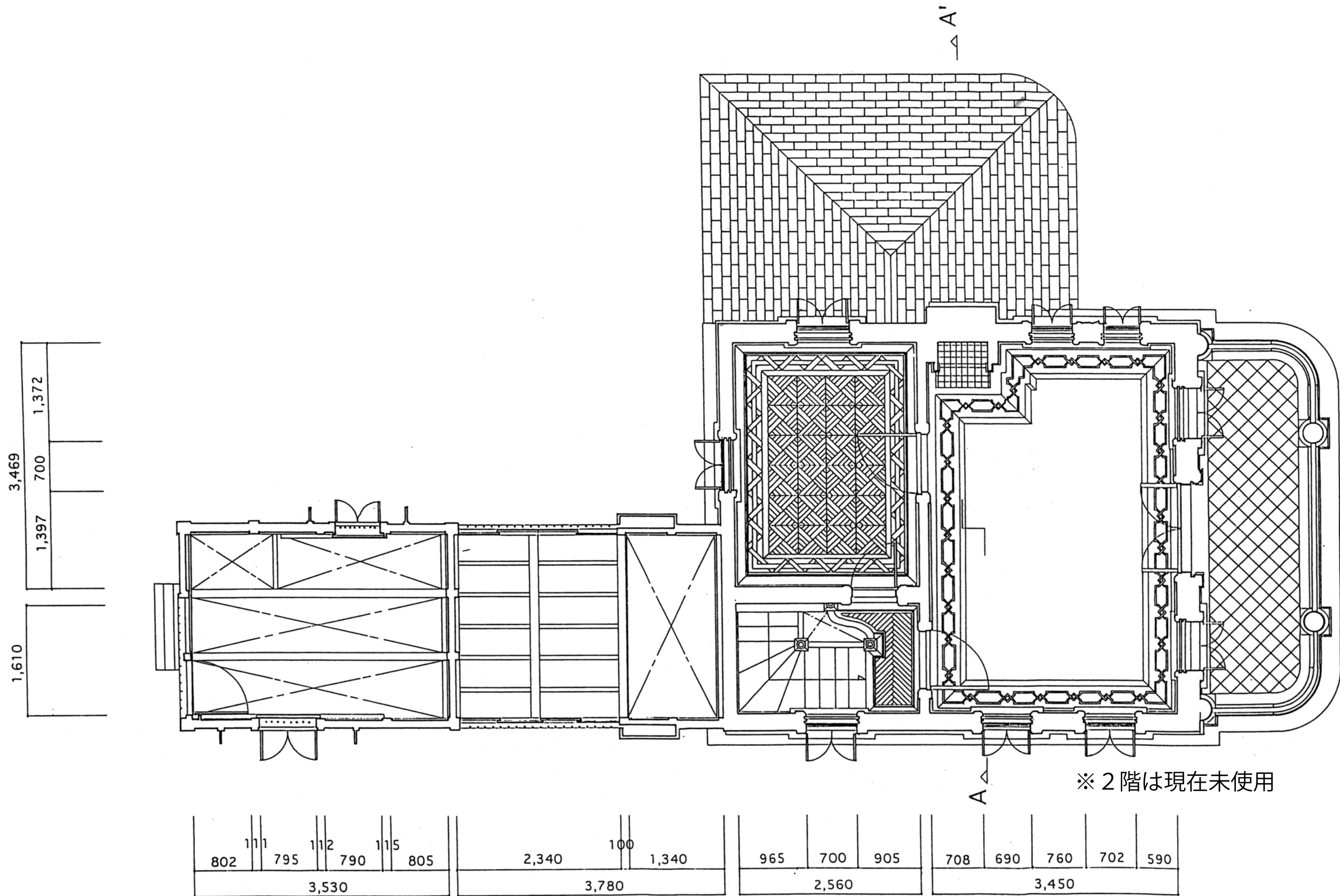
長谷子ども会館 2階平面図 (文化財部分) (S=1/50(A3))
