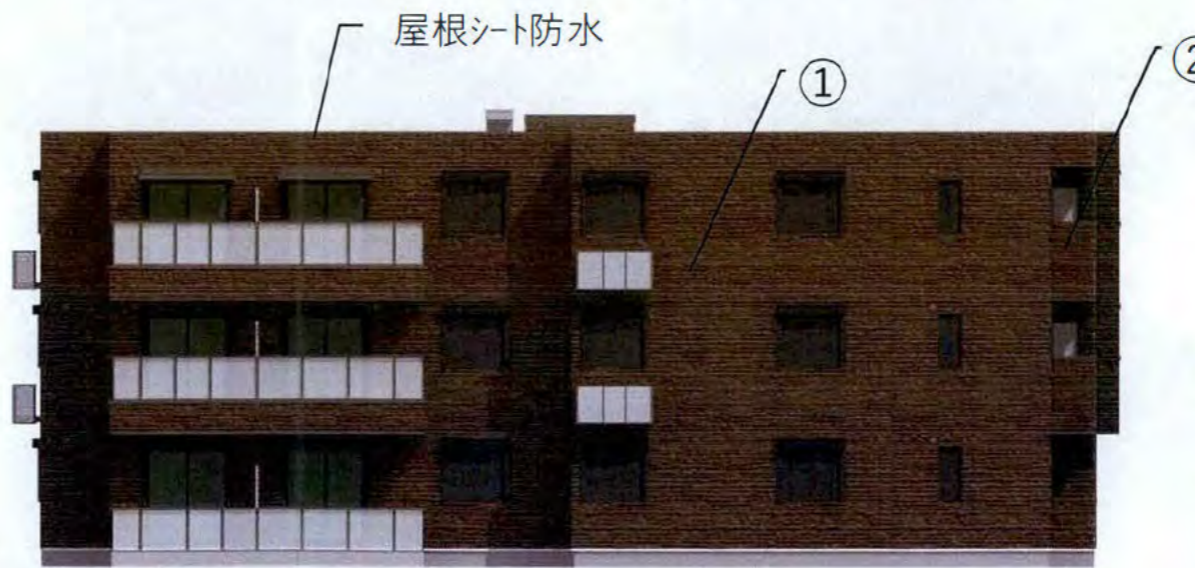
南立面図 1/150
