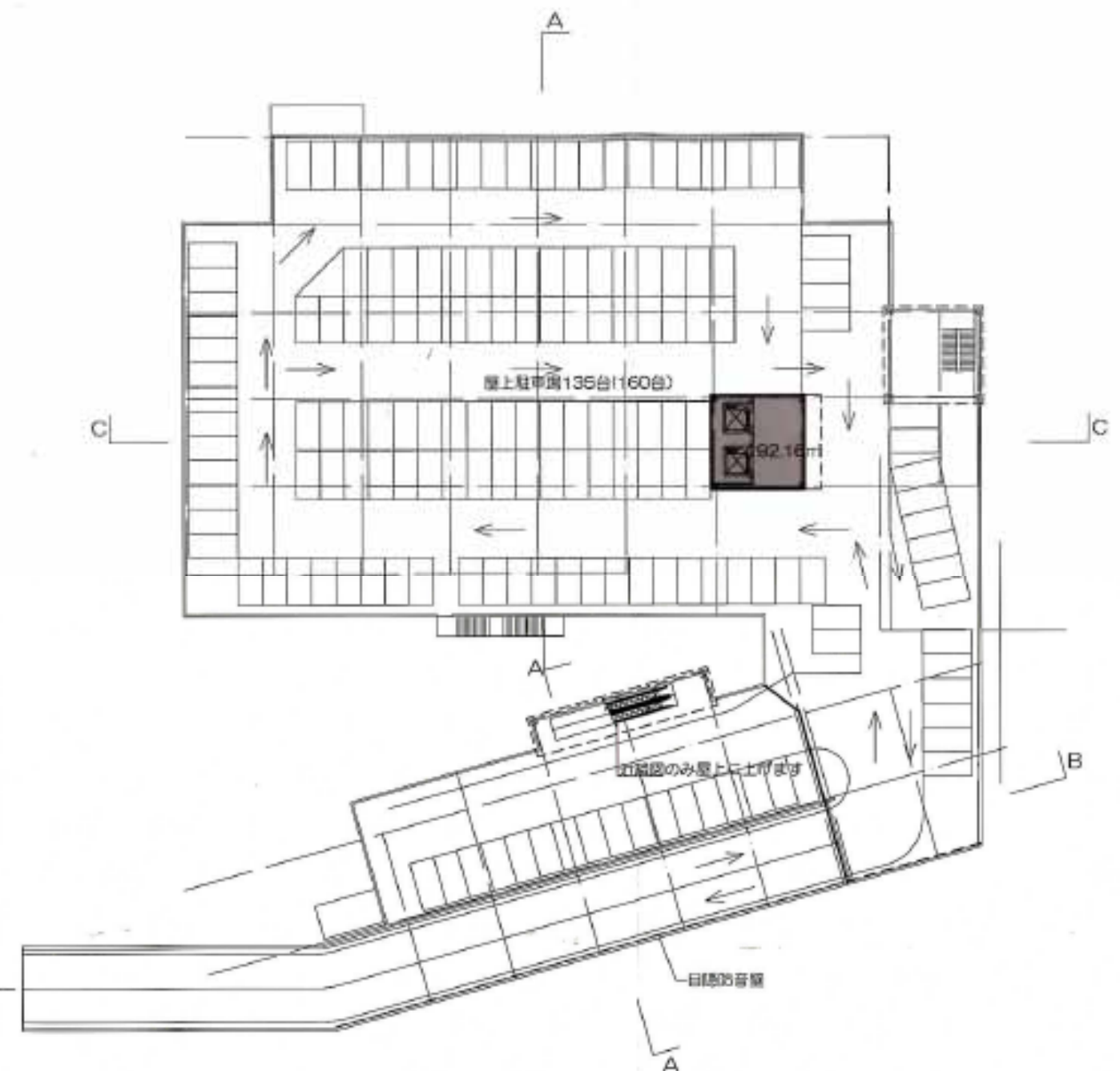
屋上階平面図
