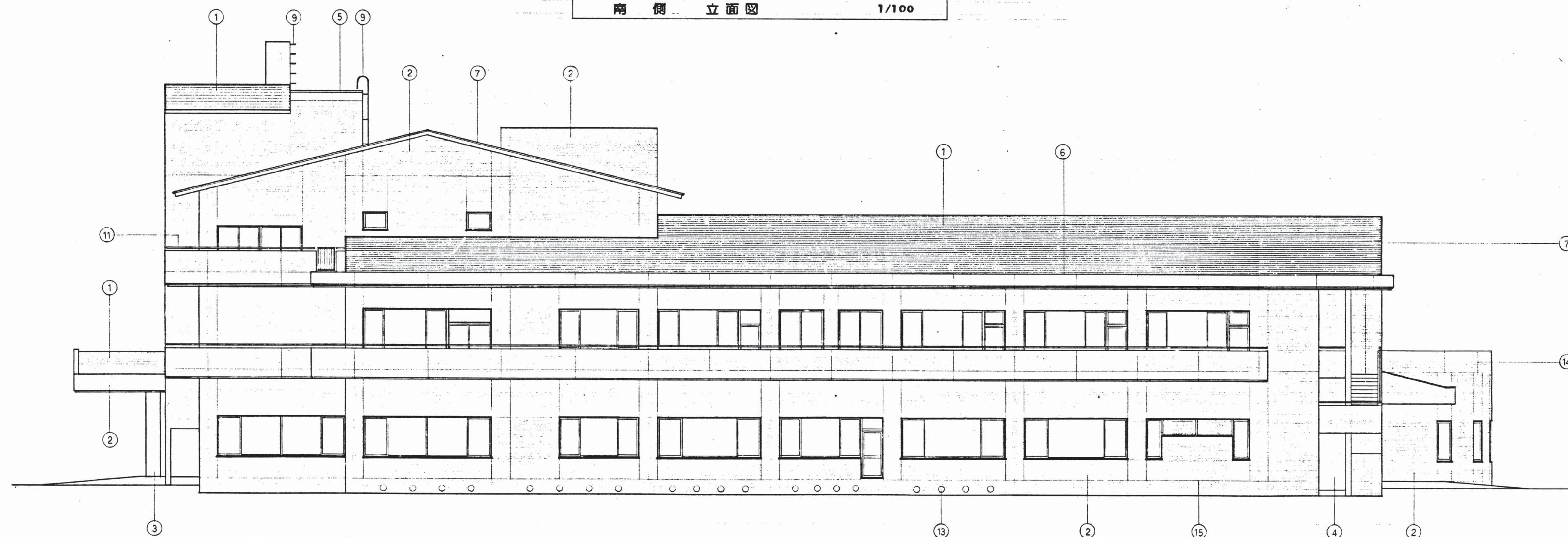
南 側 立 面 図
