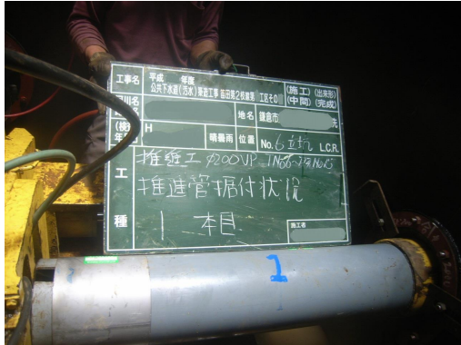
推進管(塩ビ管)掘進
