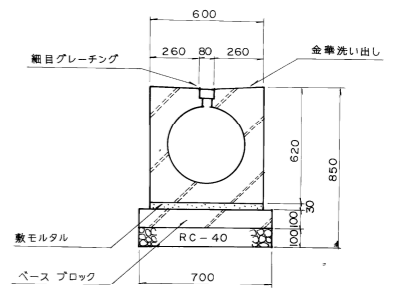
管渠型側溝 S=1/20 (φ400mm)
