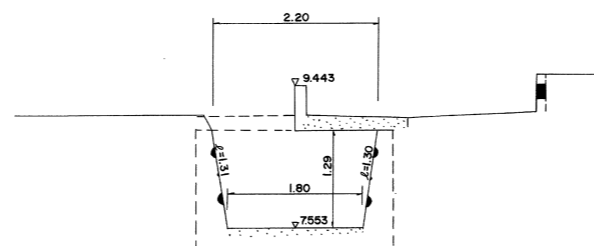
第1幹線 NO.41+5.15 GH=7.553
