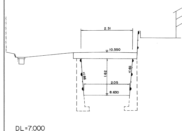
第1幹線 NO.50 GH=8.630
