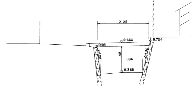
第1幹線 NO.45 GH=8.365
