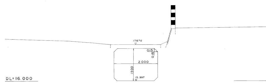
倉久保川雨水幹線 NO. 46 GH=15.997
