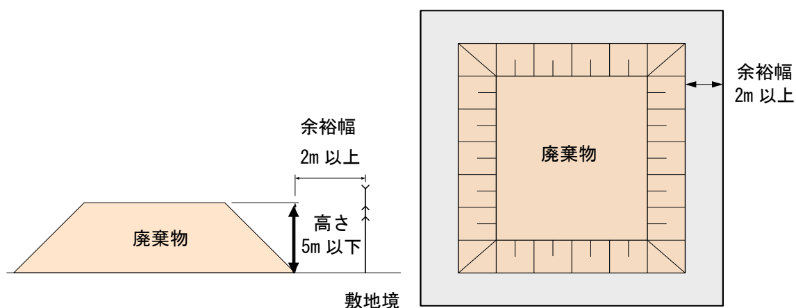
図表 2-1-17 仮置場モデル図
