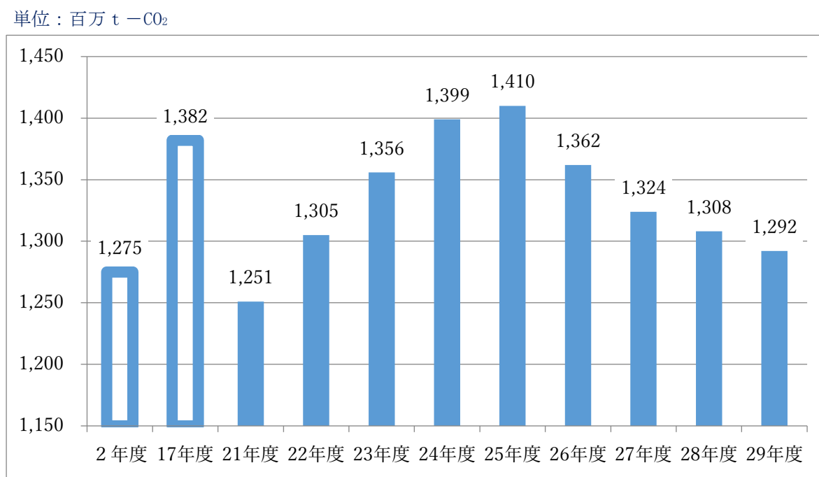
グラフ 1-2 わが国の温室効果ガス排出量の推移
