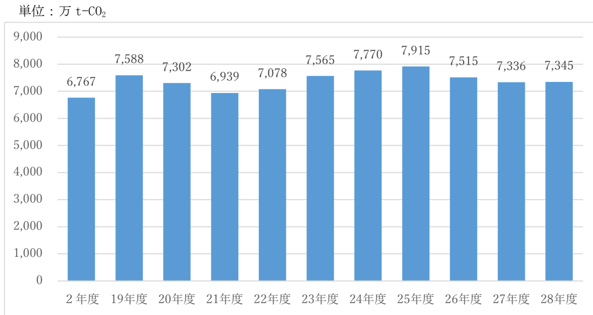
グラフ 1-3 神奈川県の二酸化炭素排出量の経年変化
