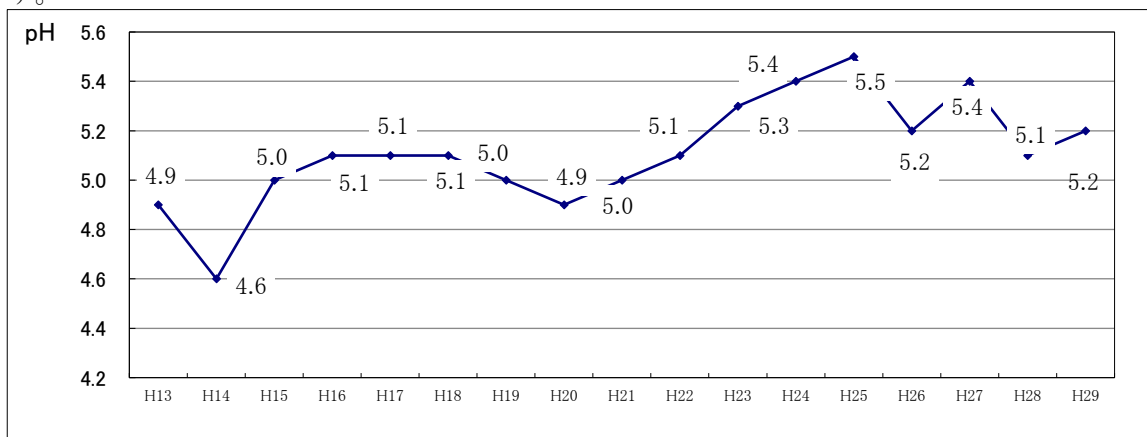
グラフ 1-5 pH測定結果
