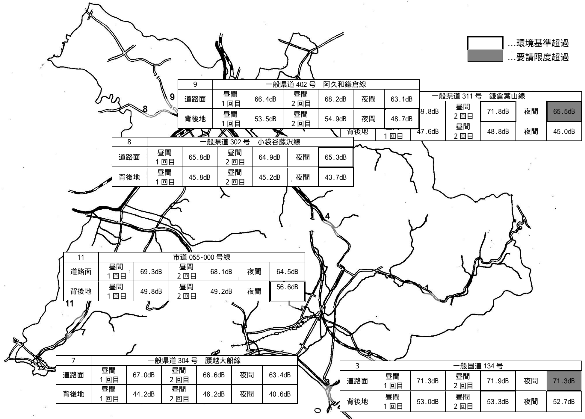
平成 21 年度 道路交通騒音状況分布図
