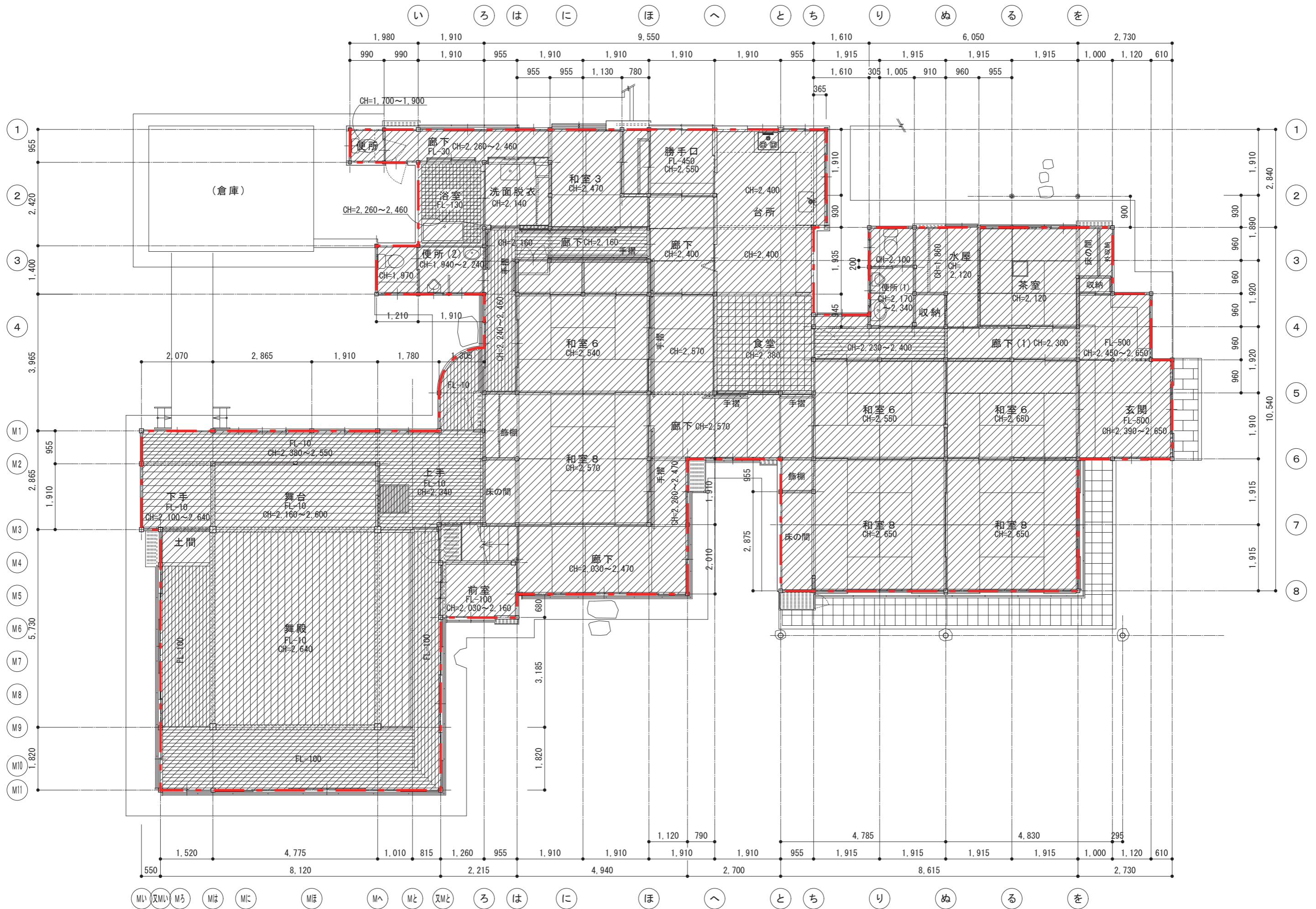
鎌倉市旧村上邸耐震診断業務委託 主屋 平面図 1階平面図
