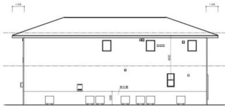
北立面図 1/100
