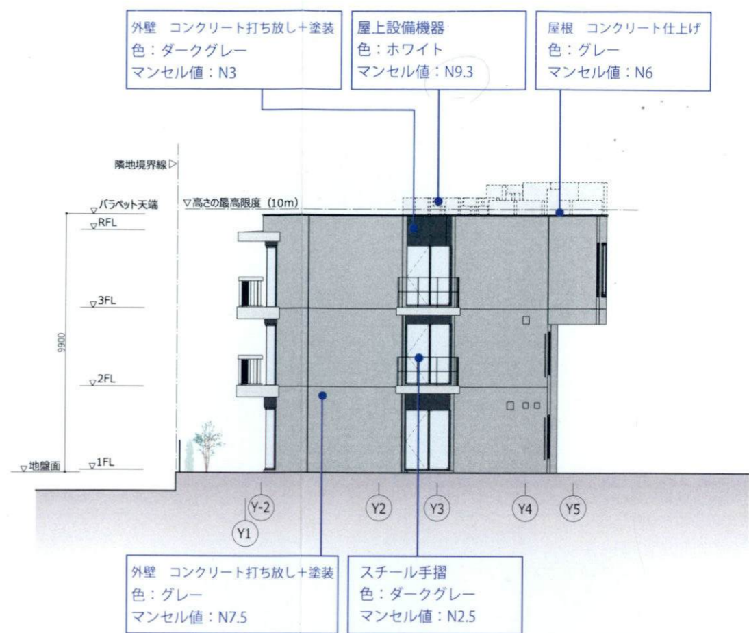
東立面図 1/200
