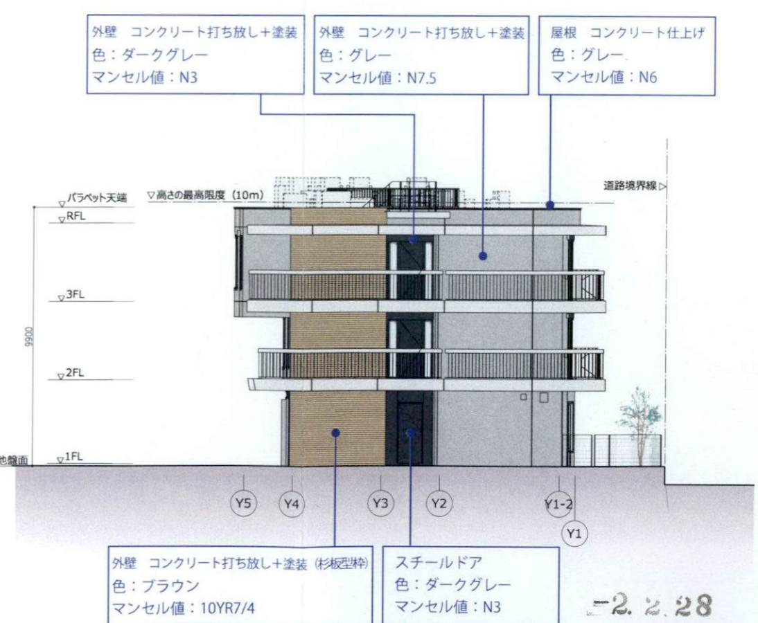
西立面図 1/200
