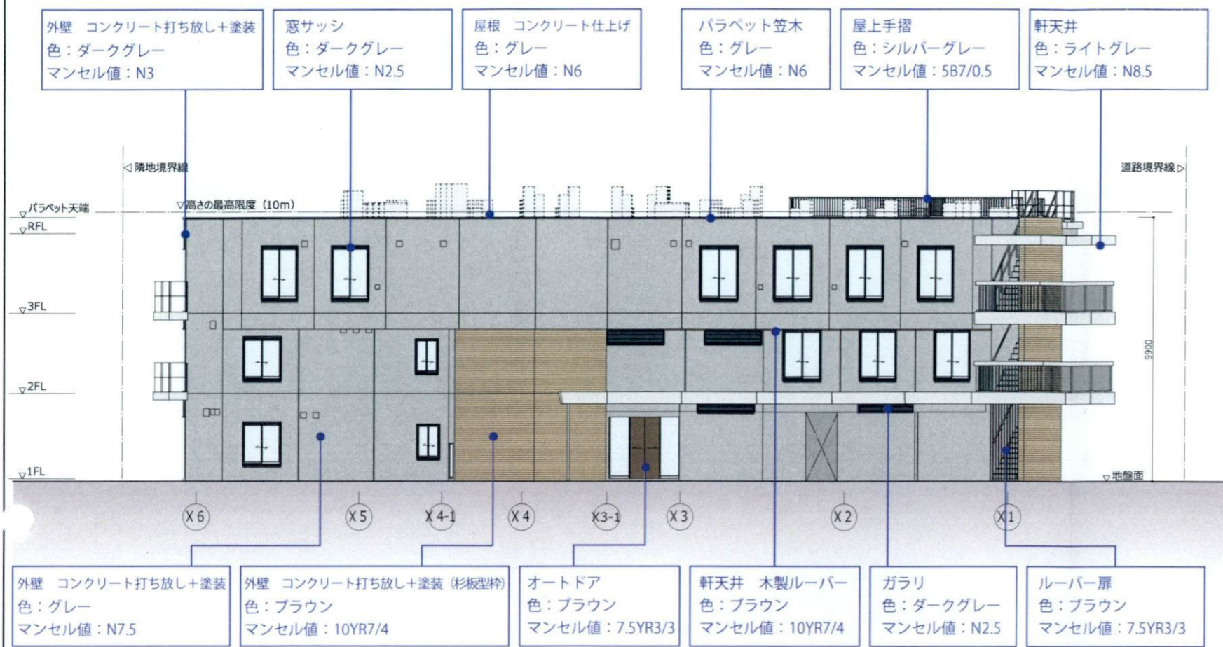
北立面図 1/200
