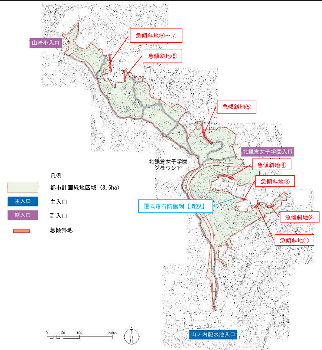
図3.5.1 落石防護網配置計画図
