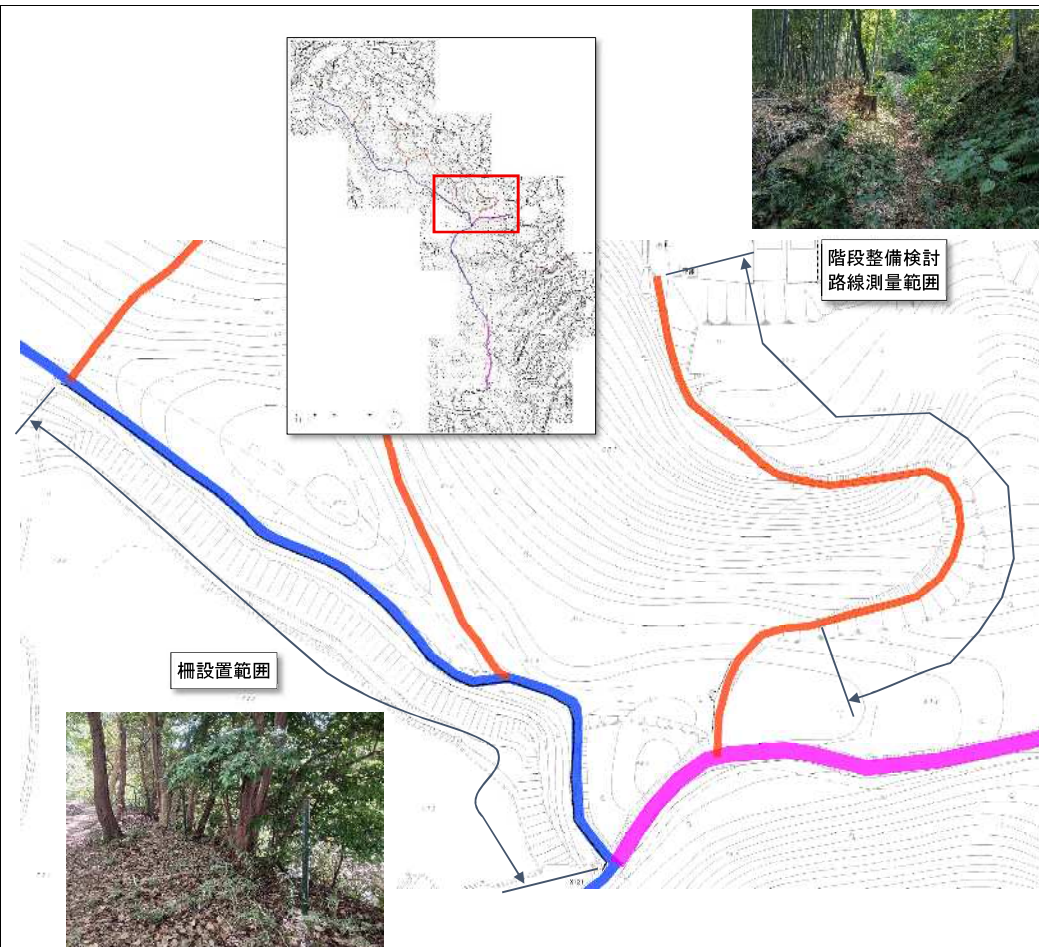
図3.3.1 階段・転落防止柵の整備箇所
