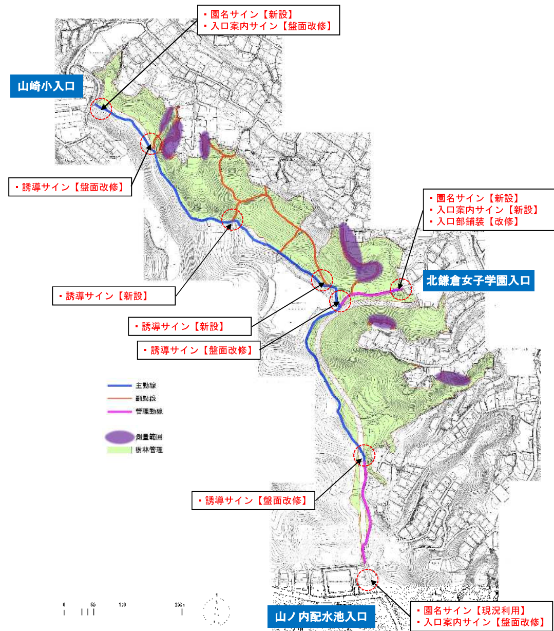
図3.6.1 全体計画図
