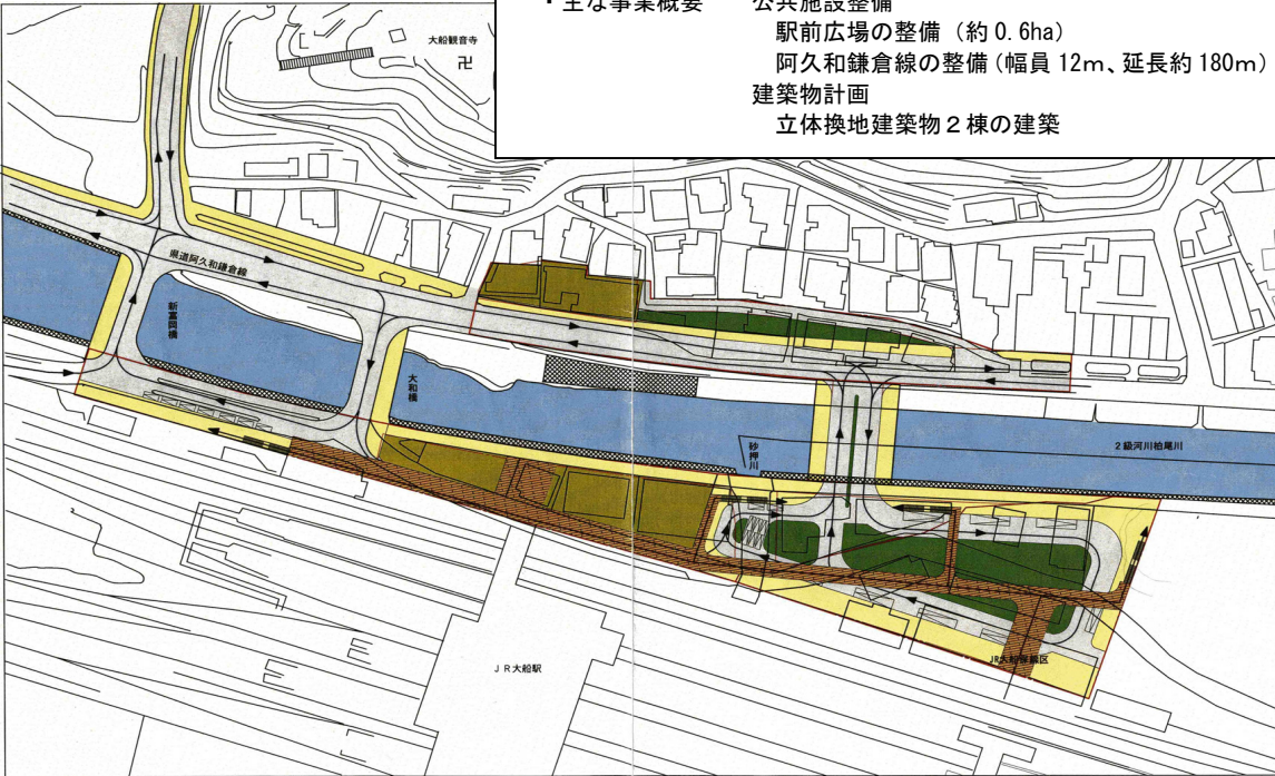
注1 横浜・鎌倉両市一体整備計画（案）
