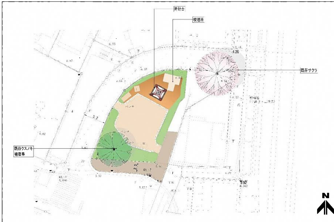
図3 現況図
