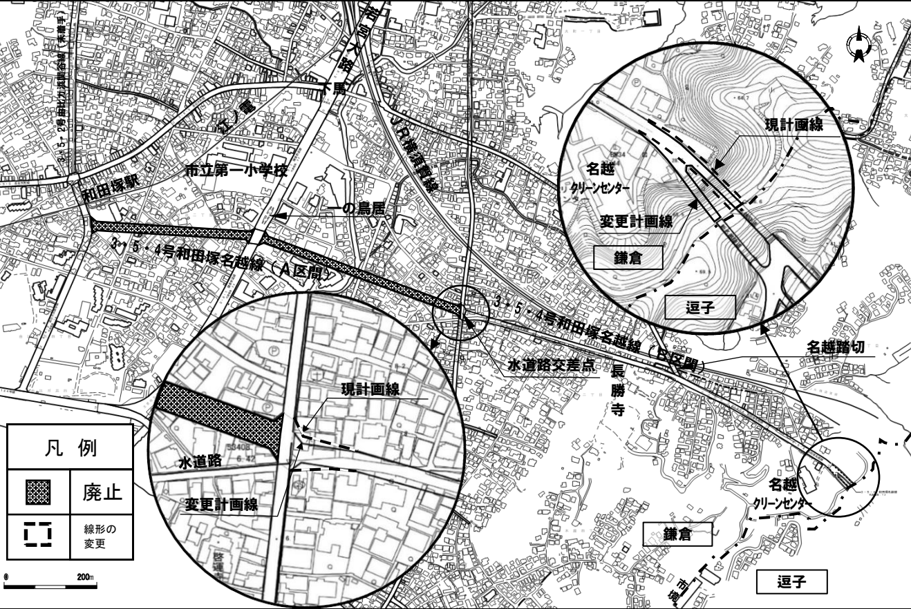
3・5・4号和田塚名越線…区間廃止・一部線形の変更
