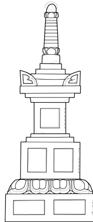
図6 極楽寺無銘宝篋印塔トレース図 (S=1/10)
