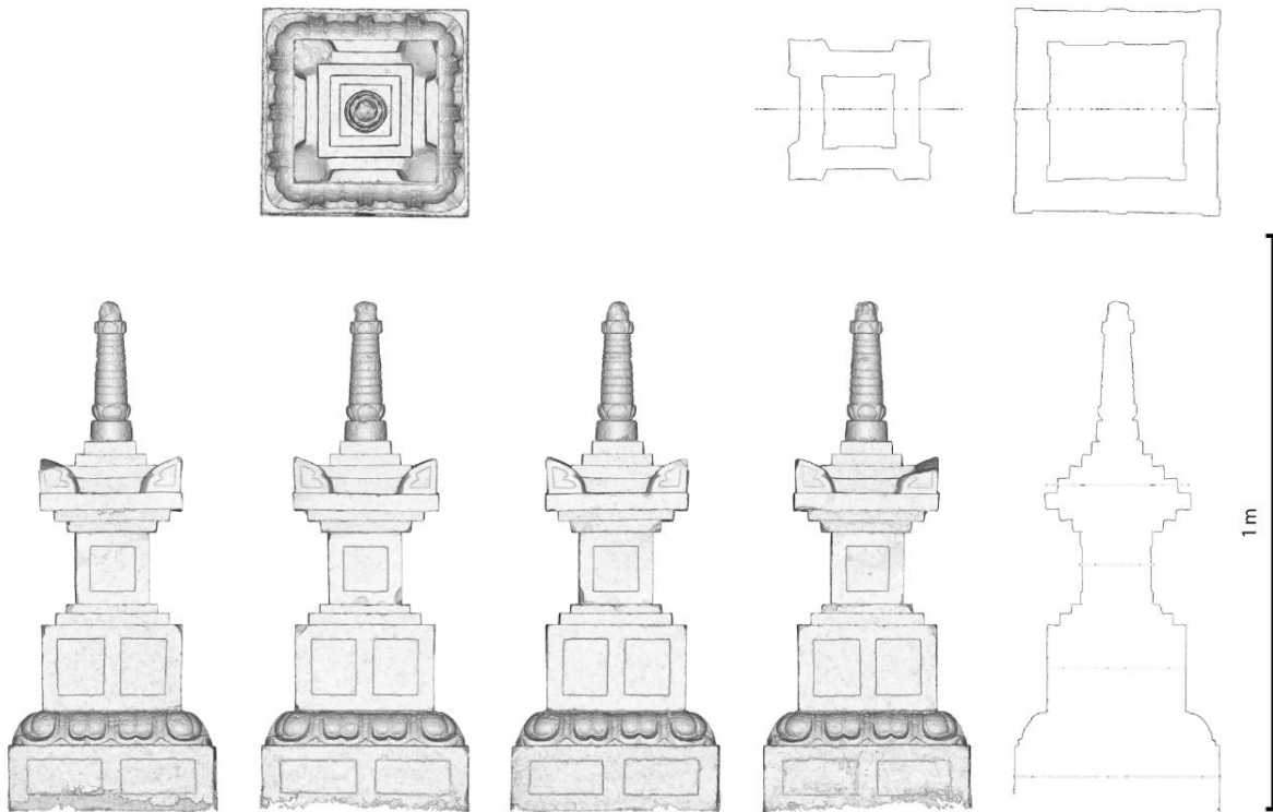
図7 極楽寺無銘宝篋印塔オルソ陰影図 (S=1/15)
