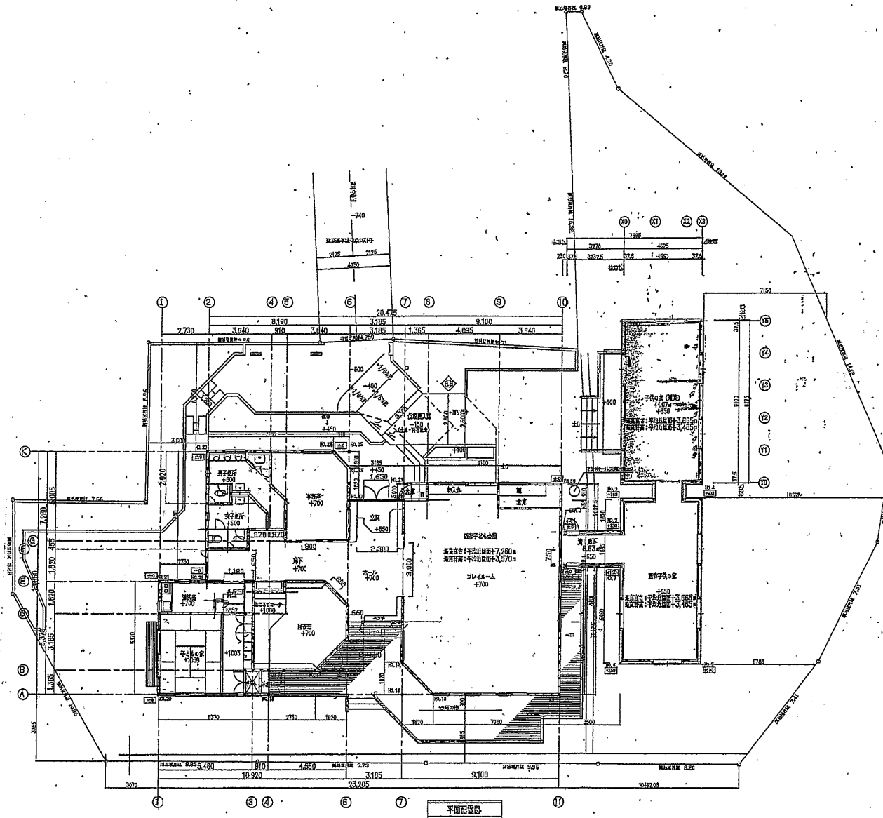
平面配置図
