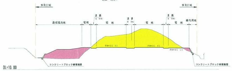
No. 6 盛土 320m 2 切土 950m 2
