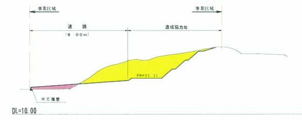
No. 2 盛土 50m 2 切土 510m 2
