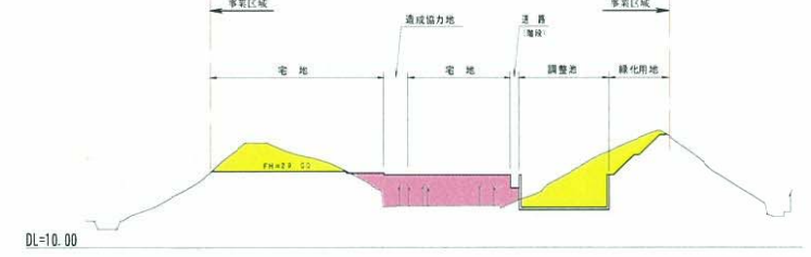
No. 10 盛土 270m 2 切土 350m 2
