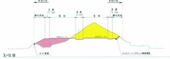
No. 7 盛土 210m 2 切土 500m 2
