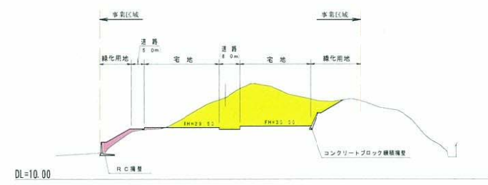
No. 8 盛土 38m 2 切土 620m 2
