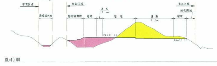
No. 5 盛土 210m 2 切土 399m 2
