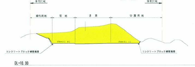
No. 3 盛土 0m 2 切土 1150m 2
