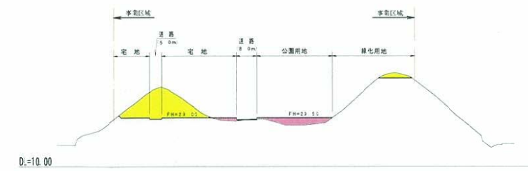
No. 9 盛土 70m 2 切土 260m 2
