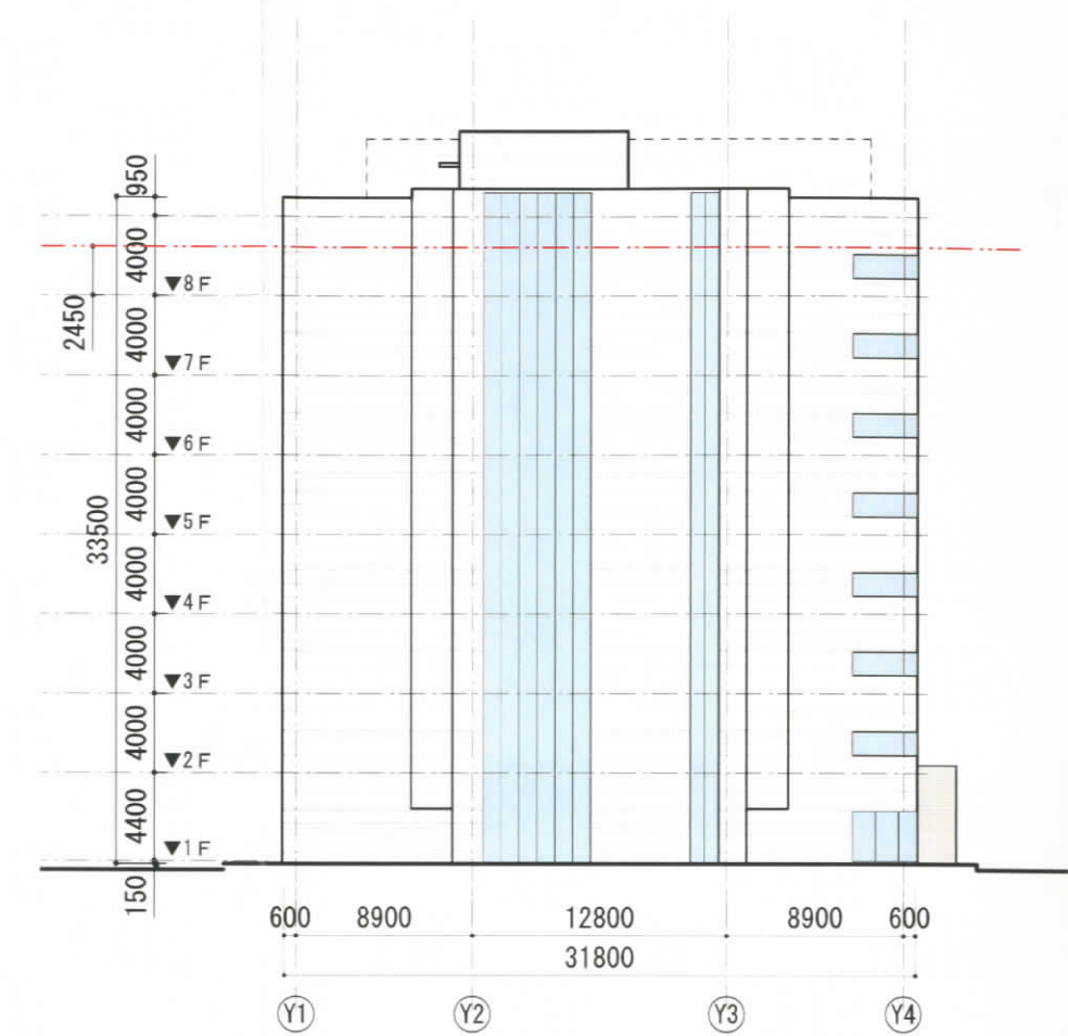
南立面図
