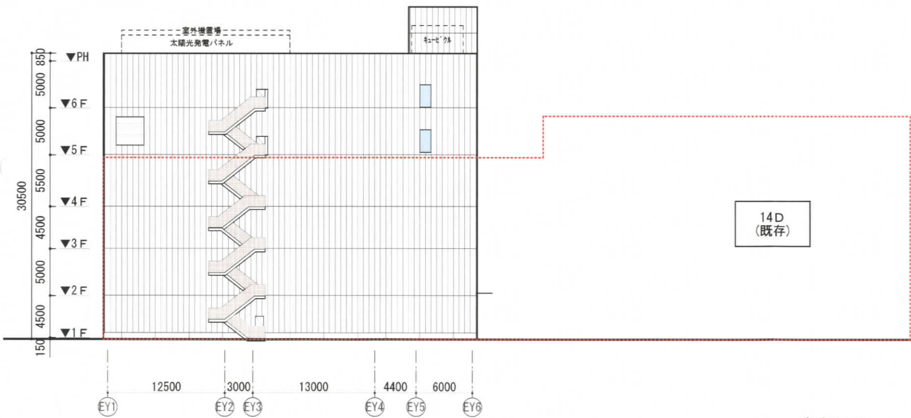
東立面図
