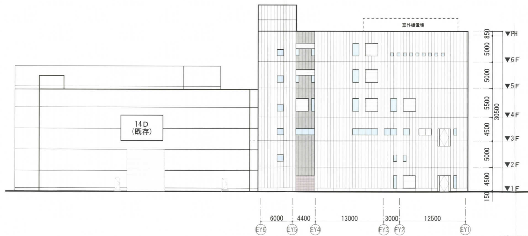
西立面図
