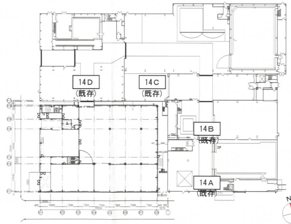
14工場1Fキープラン
