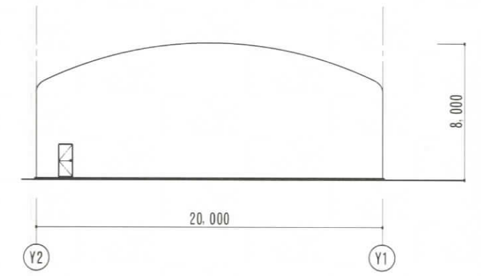
東側立面図
