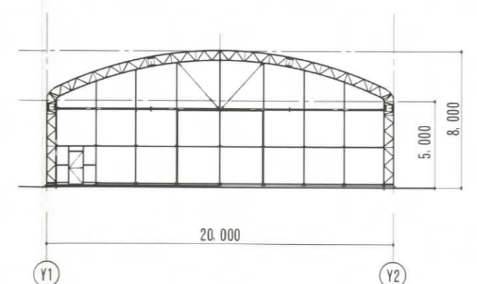
断面図 2
