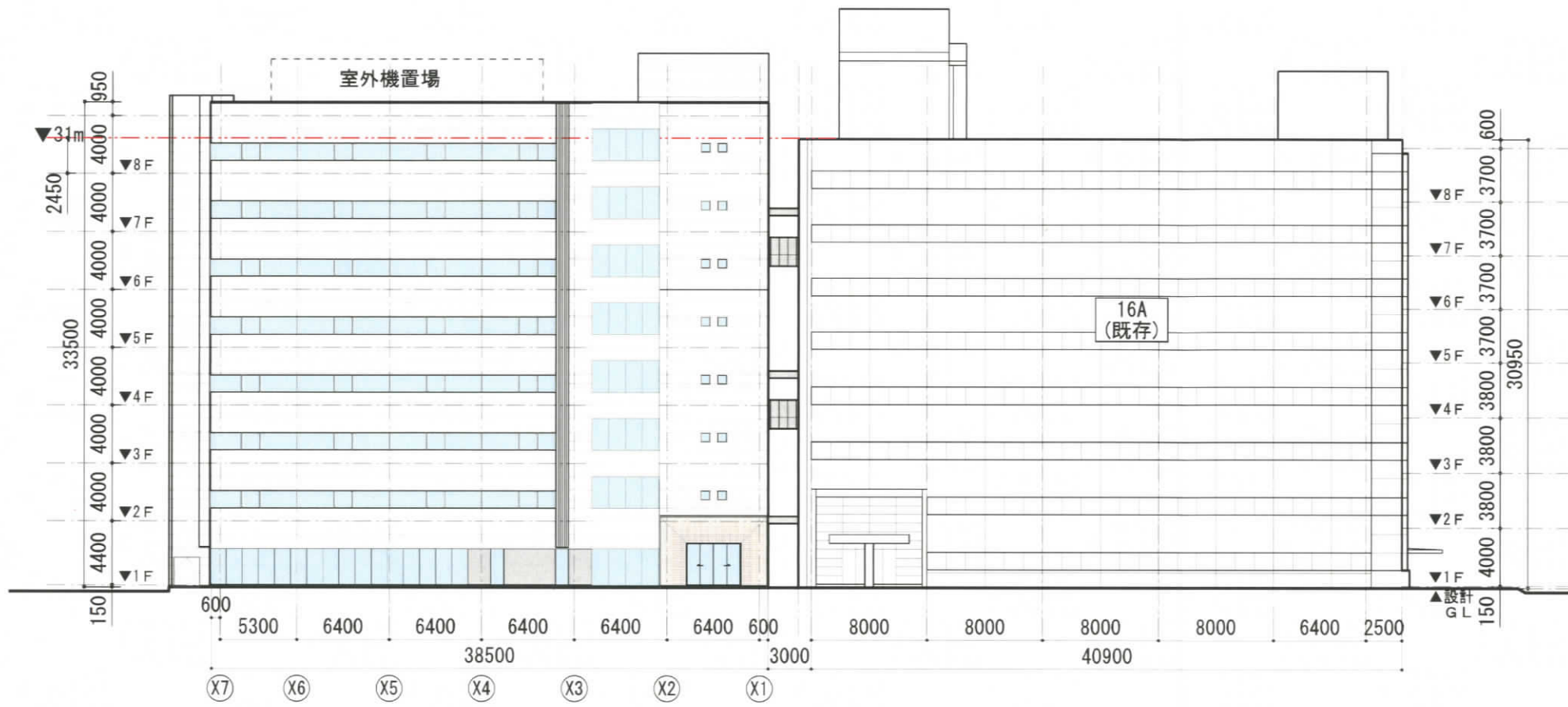
東立面図
