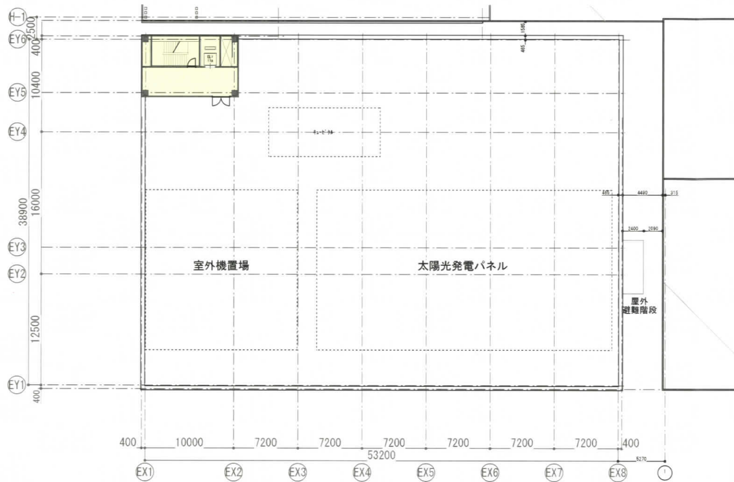
RF平面図
