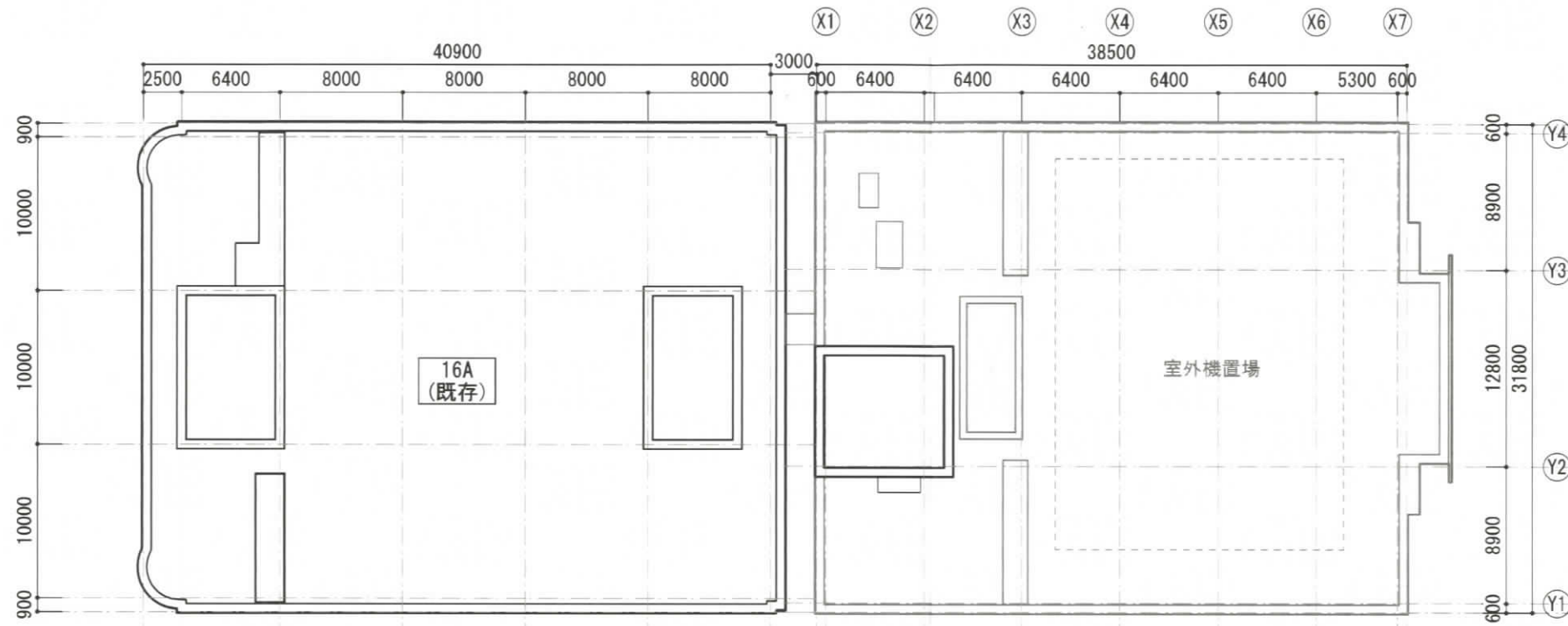
屋根伏図
