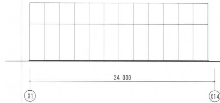
北側立面図
