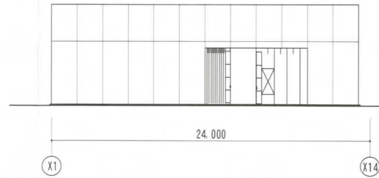
南側立面図
