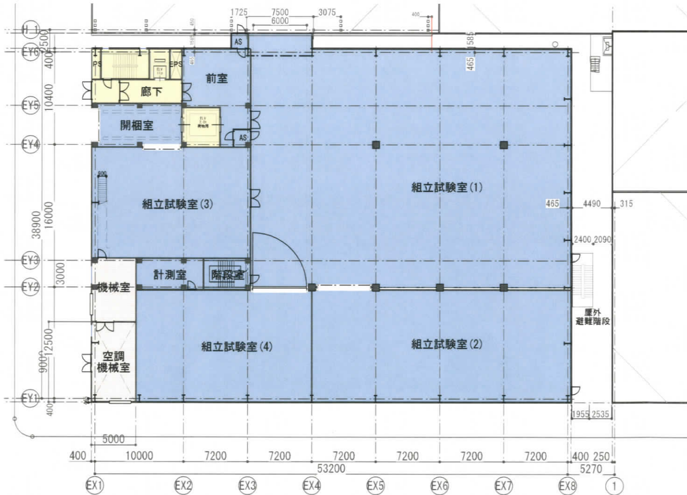
2階平面図
