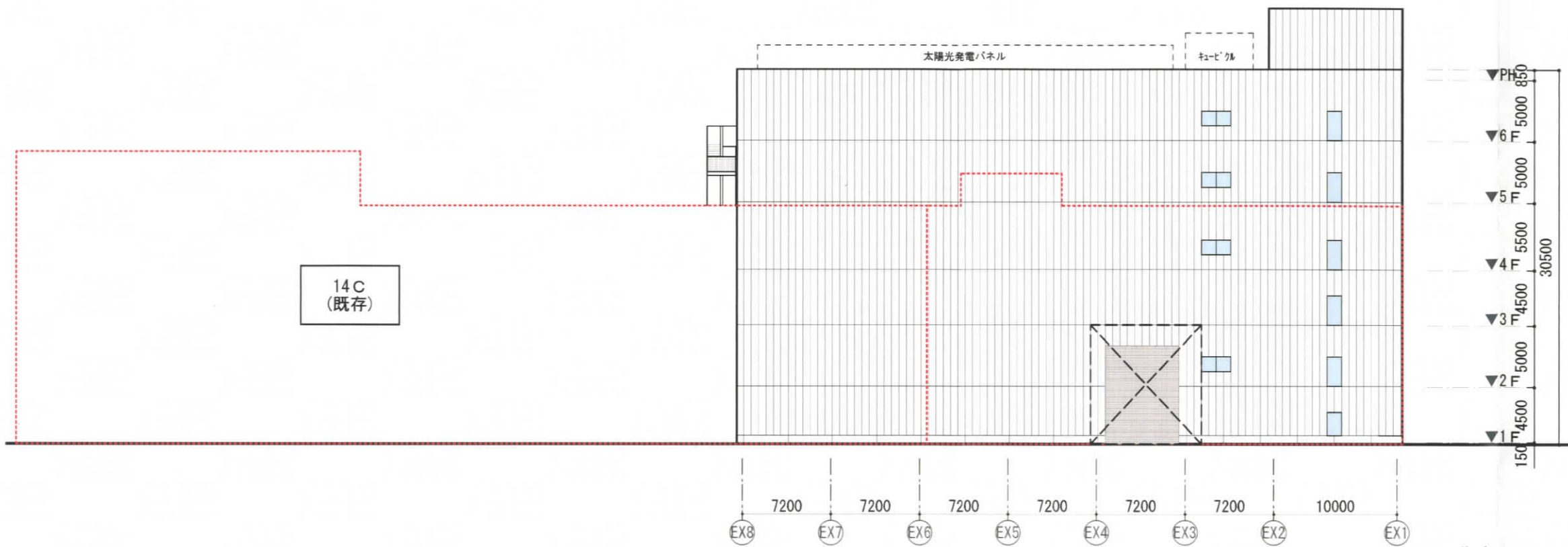
北立面図
