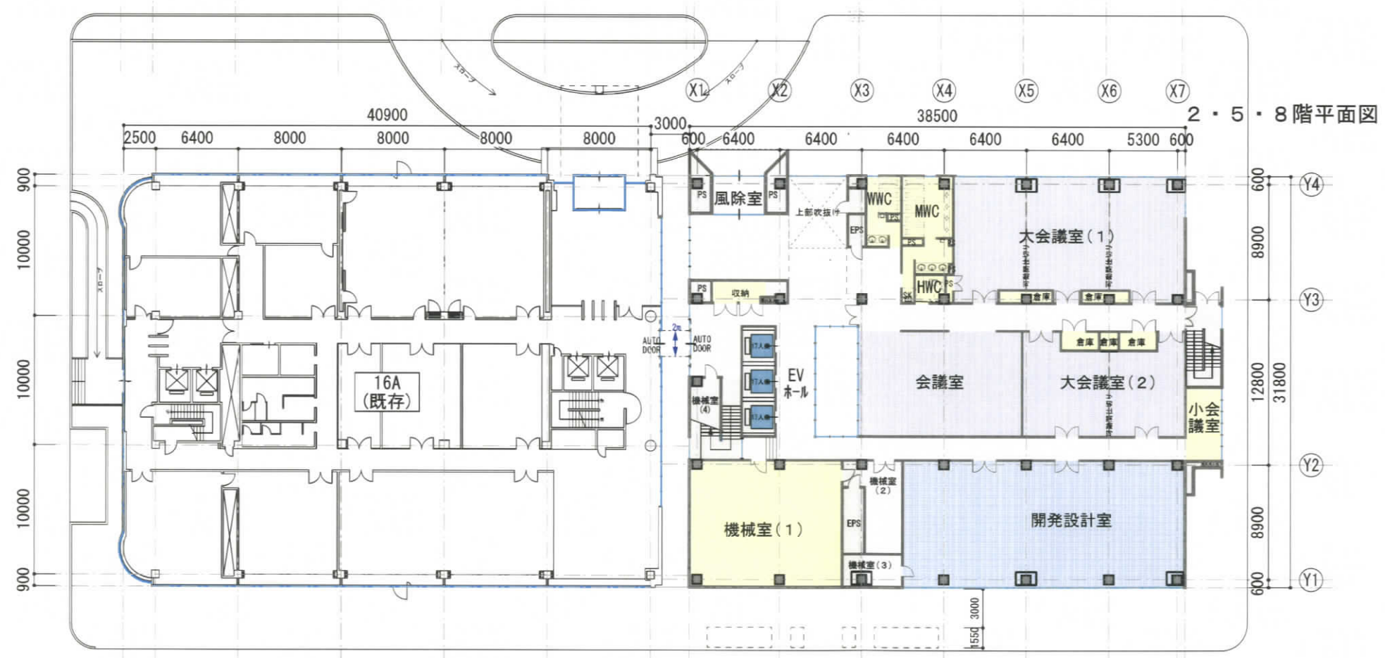
1階平面図 16B工場
