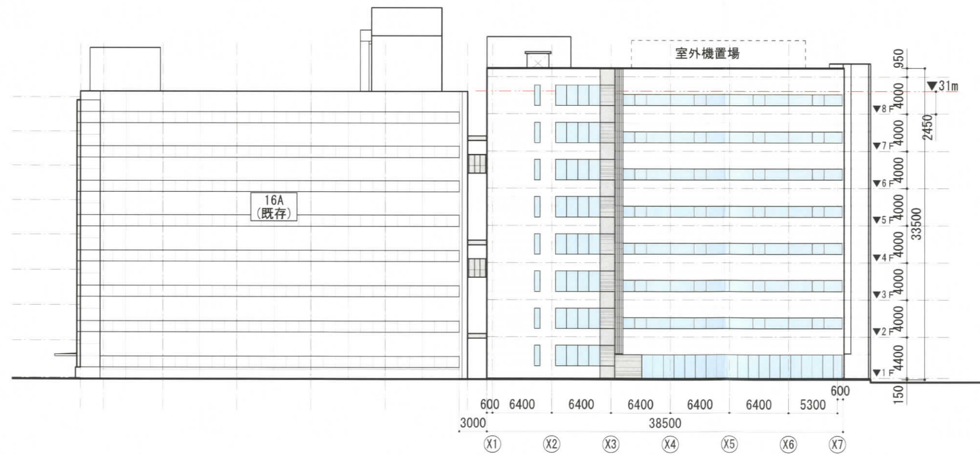
西立面図
