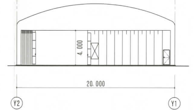
西側立面図
