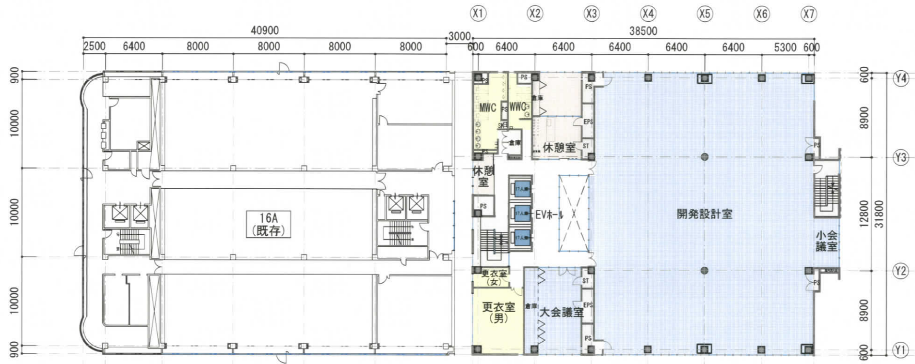
4階平面図
