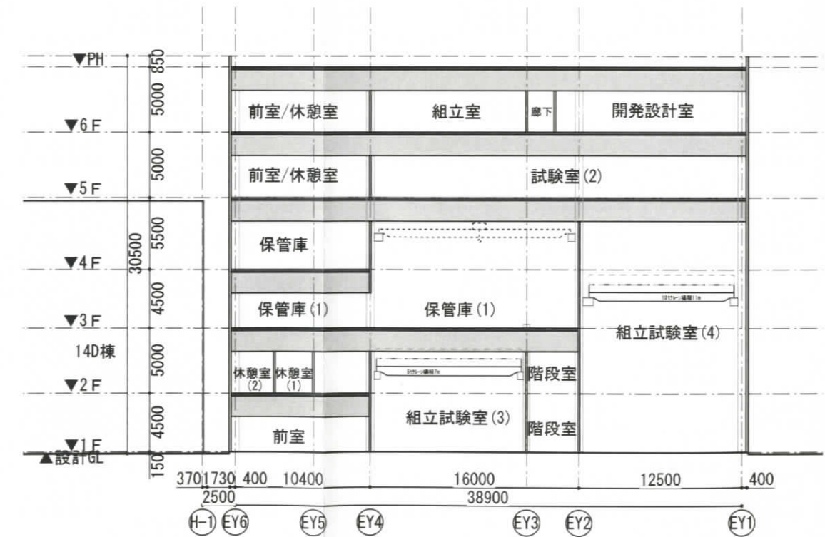
A-A' 断面図
