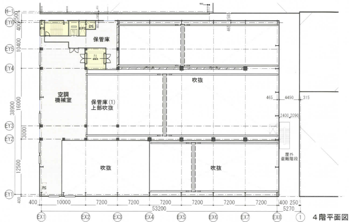
4階平面図
