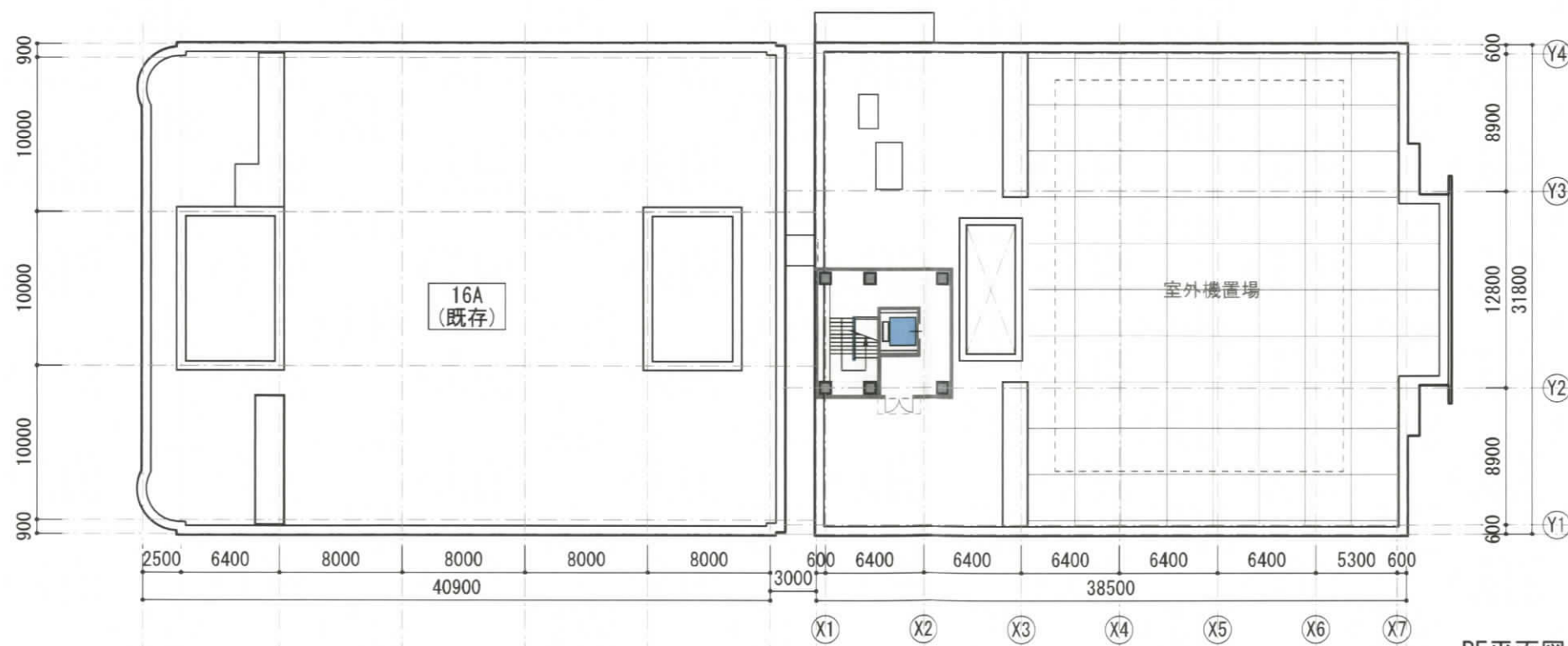
RF平面図
