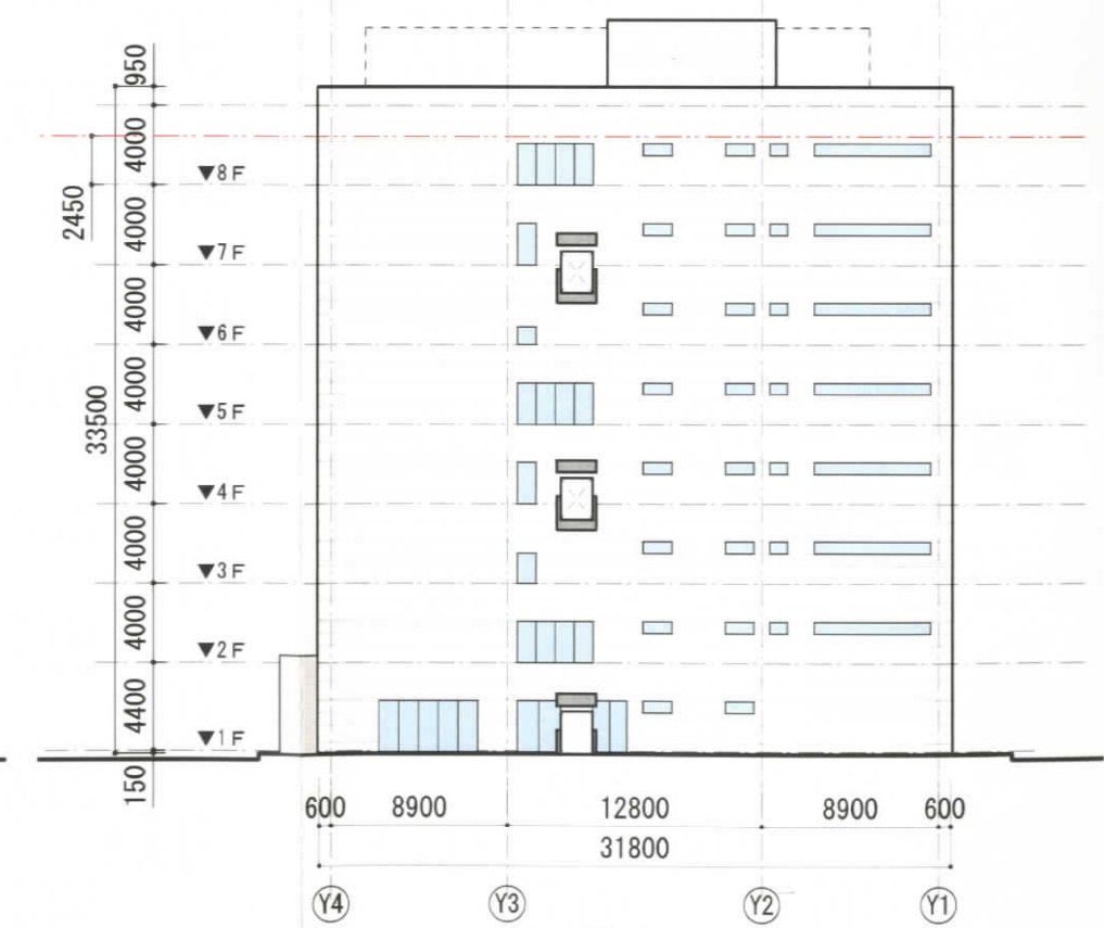
北立面図
