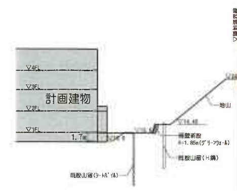
C断面図
