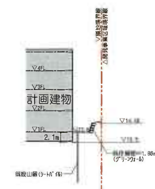
D断面図
