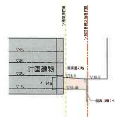
E断面図
