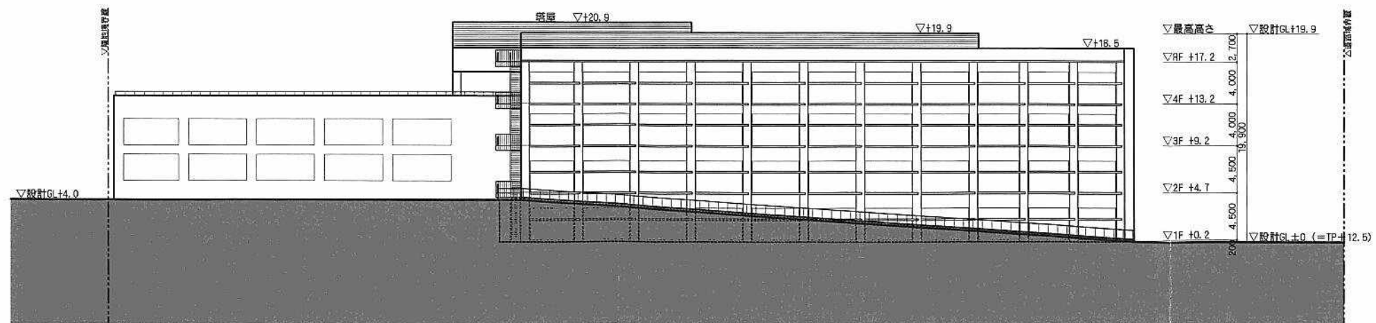
東立面図
