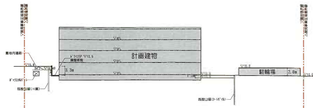
A断面図
