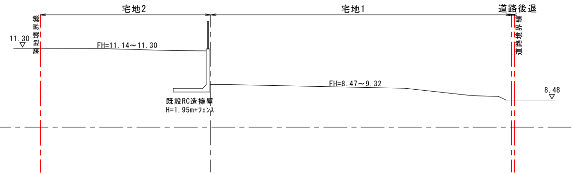
⑫ - ⑫ 断面
