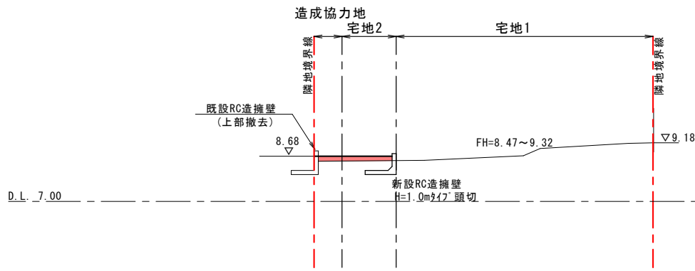
⑮ - ⑮ 断面
