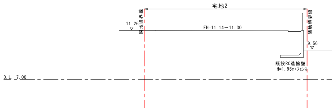
⑬ - ⑬ 断面
