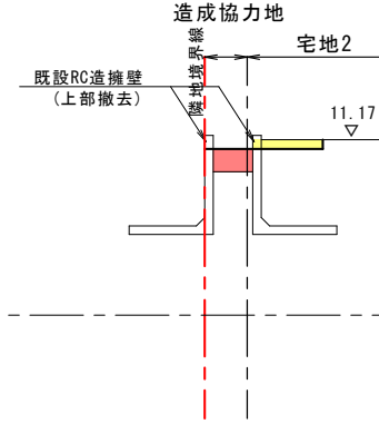
⑯ 断面
