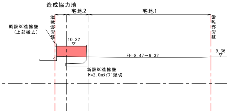
⑭ - ⑭ 断面
