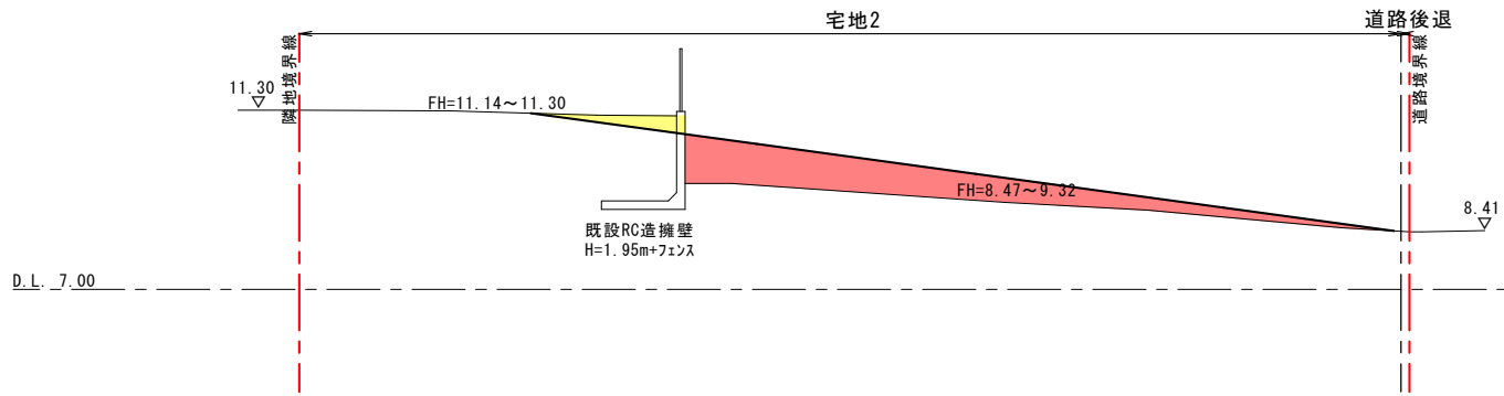
⑪ - ⑪ 断面
