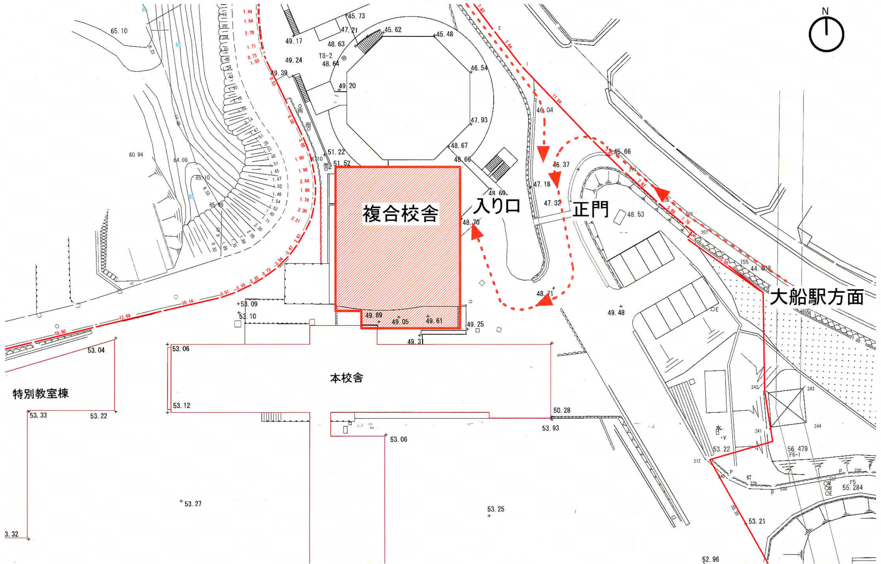
配置図 縮尺1:400
