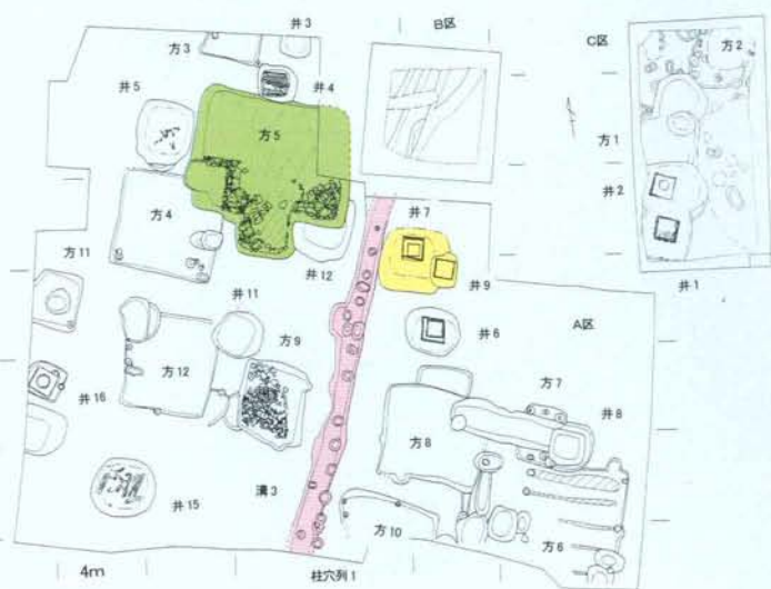
遺構配置図 (発掘調査区全景)
