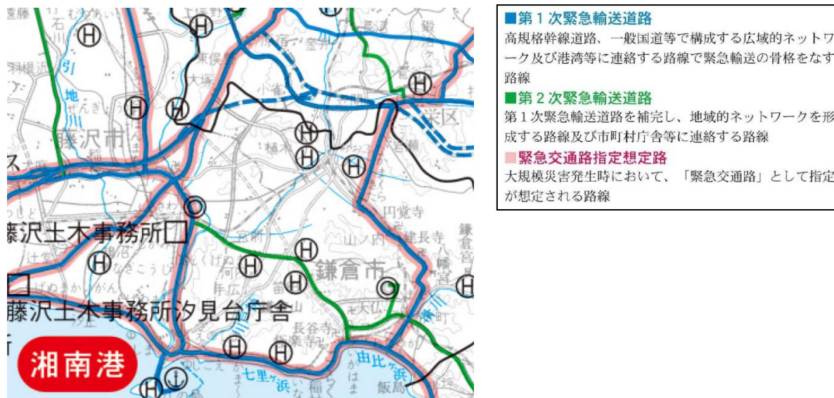
図 緊急輸送道路網図（資料：神奈川県緊急輸送道路網図（令和4年（2022年）3月））
